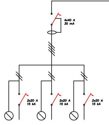
ESQUEMA DE CUADRO DE MANDO Y CENTRO DE MANDO 4
