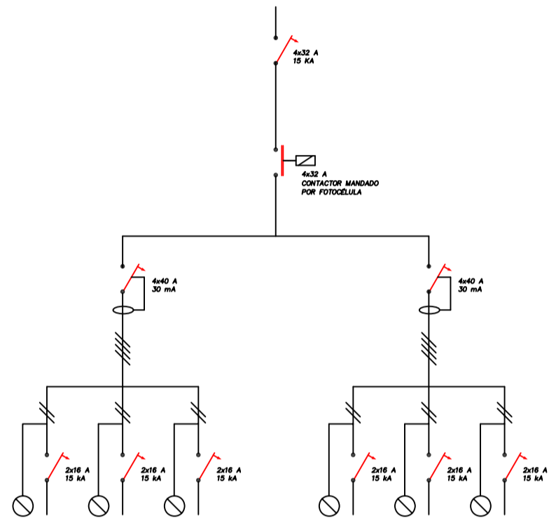
ESQUEMA DE CUADRO DE MANDO Y PROTECCION CENTRO DE MANDO 2
