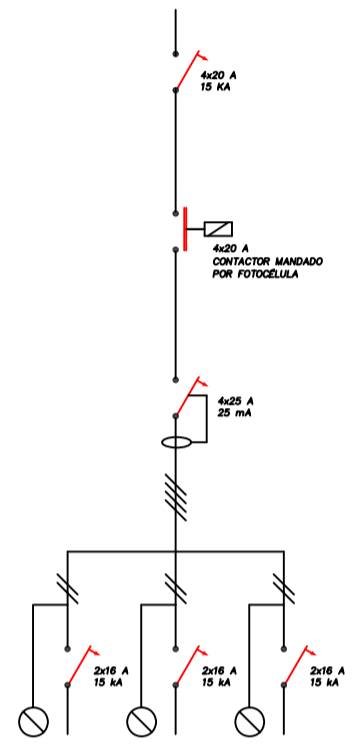
ESQUEMA DE CUADRO DE MANDO Y CENTRO DE MANDO 4
