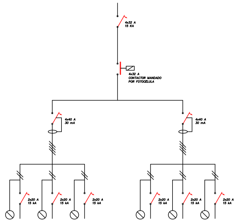
ESQUEMA DE CUADRO DE MANDO Y PROTECCION CENTRO DE MANDO 1
