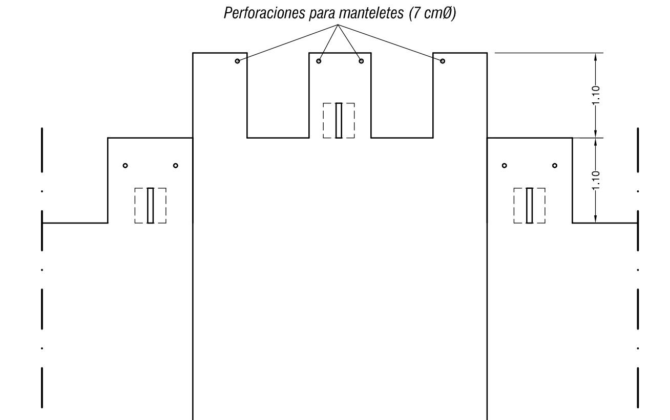
Alzado exterior
