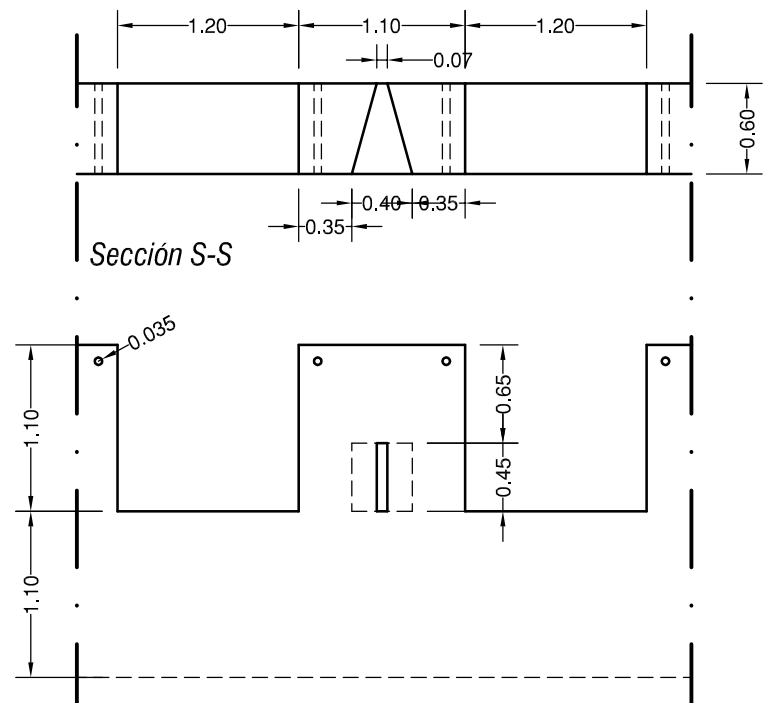
Alzado exterior
